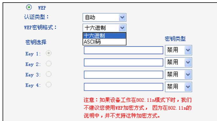
图 6-25 WEP 安全模式
