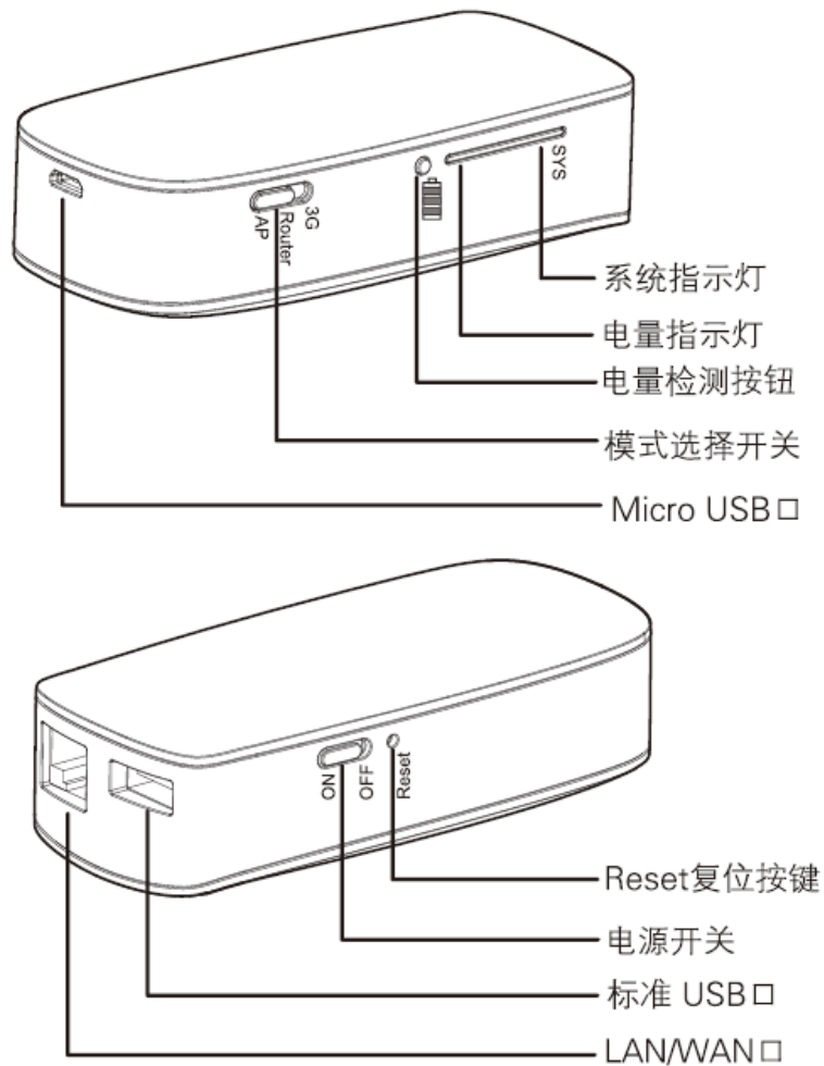
图 3-1 TL-MR12U 外观图
